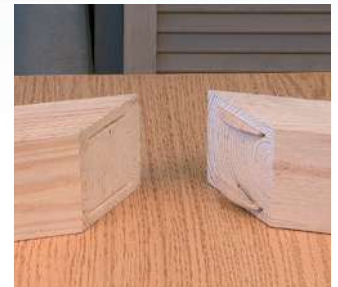
Ensamblajes de extrema solidez con pastillas grandes del No. 6.
