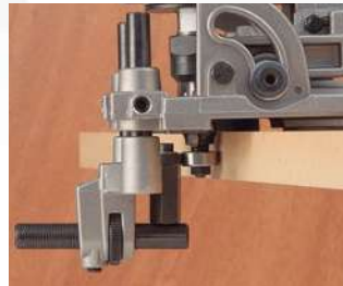
Freno del rodamiento de la fresa para evitar marcas sobre el panel.
