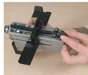
Ajuste micrométrico de la anchura de corte.
