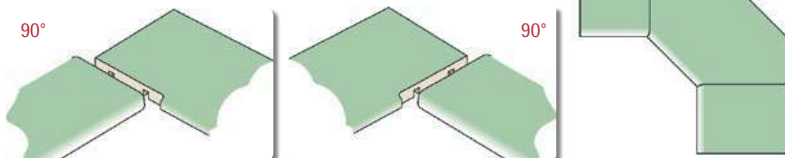
El ngulo de ensamblaje puede ser de 45° o 90°
